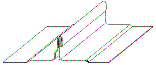
Doppelstehfalz mit Clip Relief
